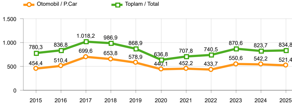
Toplam Üretim ve Otomobil Üretimi (x1000)(OCAK - TEMMUZ) Total & P.Cars Production (x1000)(January - July)
