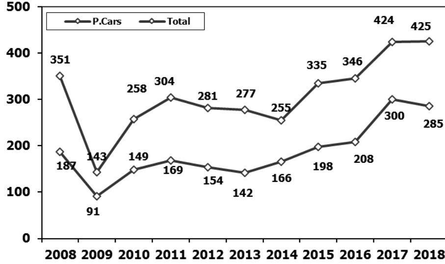
2008-2018 Toplam ve Otomobil Üretim Gelişimi (Ocak-Mart) (x1000)
